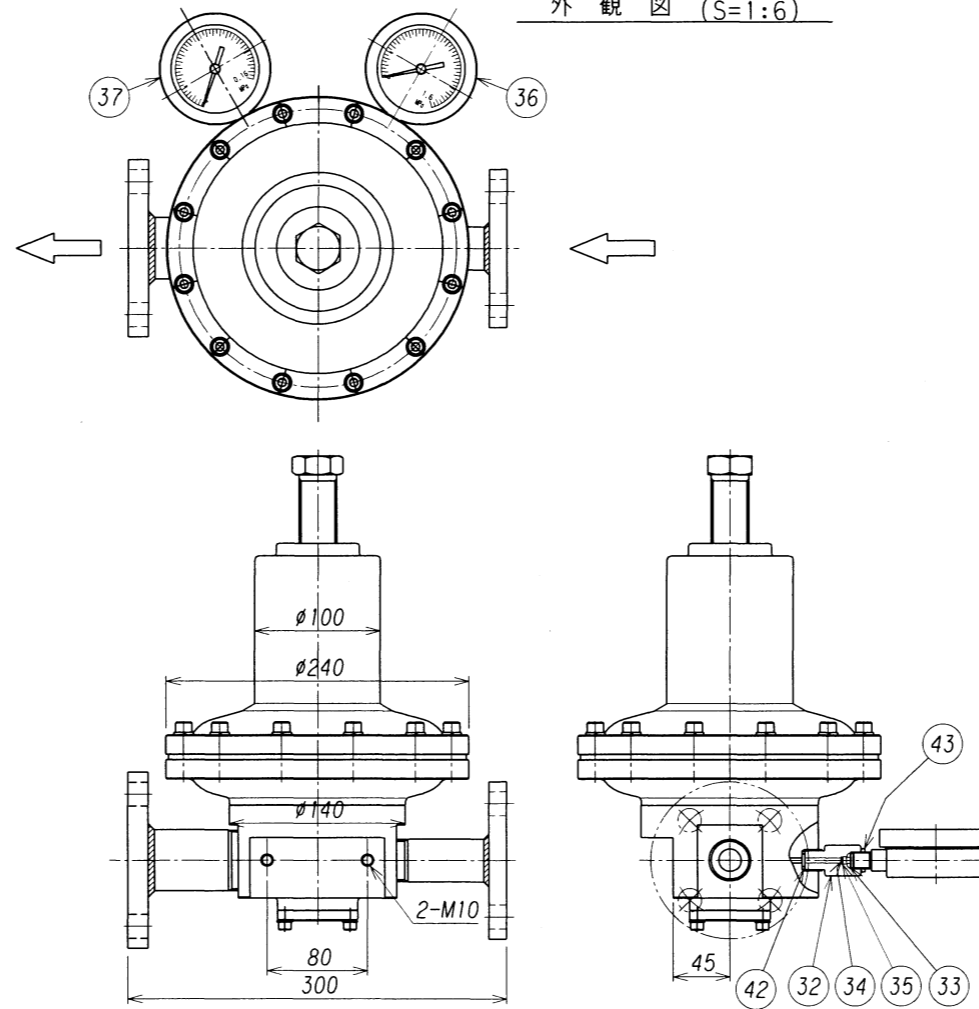
外観図 (S=1:6)
