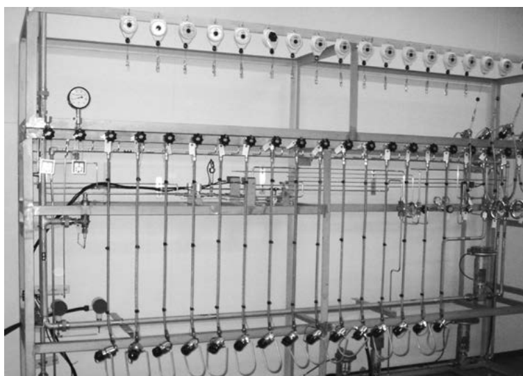
【液化酸素 (LGC) 自動充填装置 施工例】
