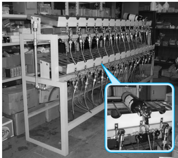
【直列式・水平型充填架台施工例】
