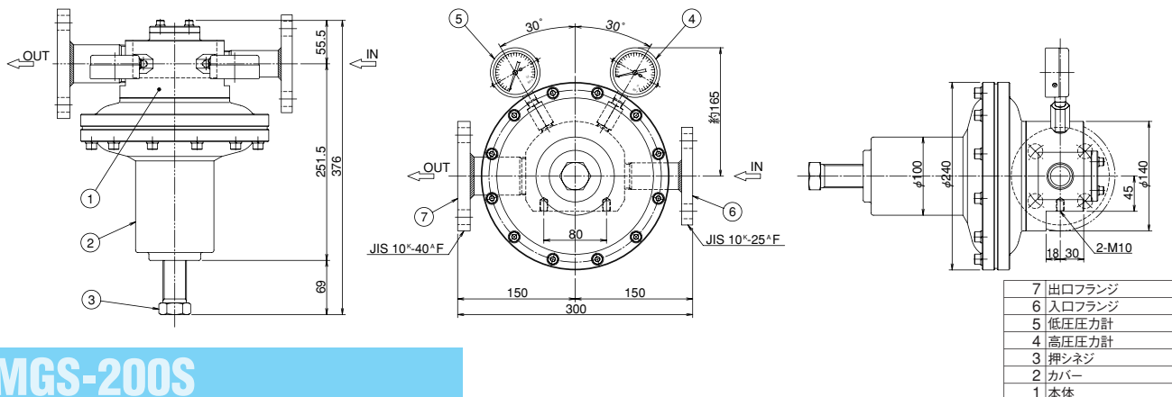
【外観寸法図】
