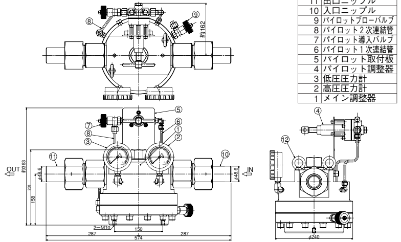
【外観寸法図】
