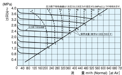
【TKR-200/TKR-200S型流量表】
