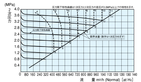
【TKR-200-H/TKR-200S-H型流量表】
