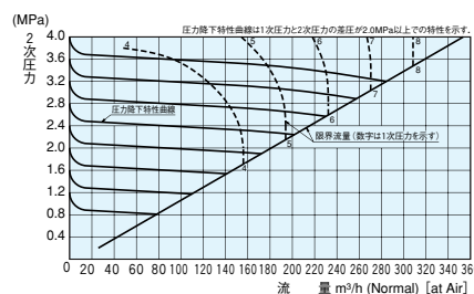
【TKR-140/TKR-140S型流量表】
