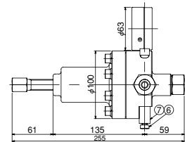
【TKR-140-H/TKR-140S-H型流量表】
