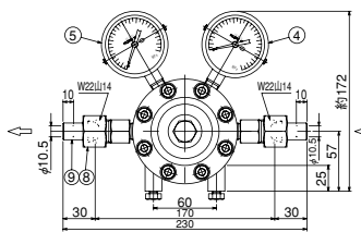
【TKR-140/TKR-140S型流量表】
