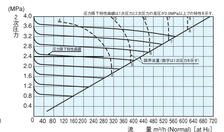
【TKR-140-H/TKR-140S-H型流量表】
