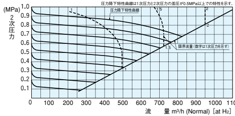
【GS-200L2-H/GS-200L2S-H型 流量表】
