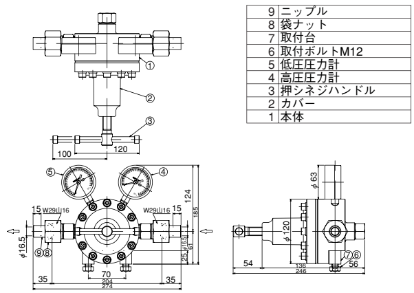
【外観寸法図】
