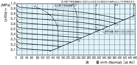
【GS-200L-H/GS-200LS-H型 流量表】
