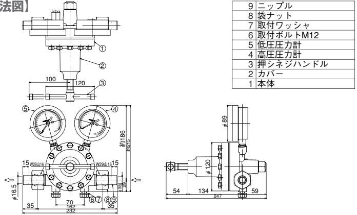
【外観寸法図】
